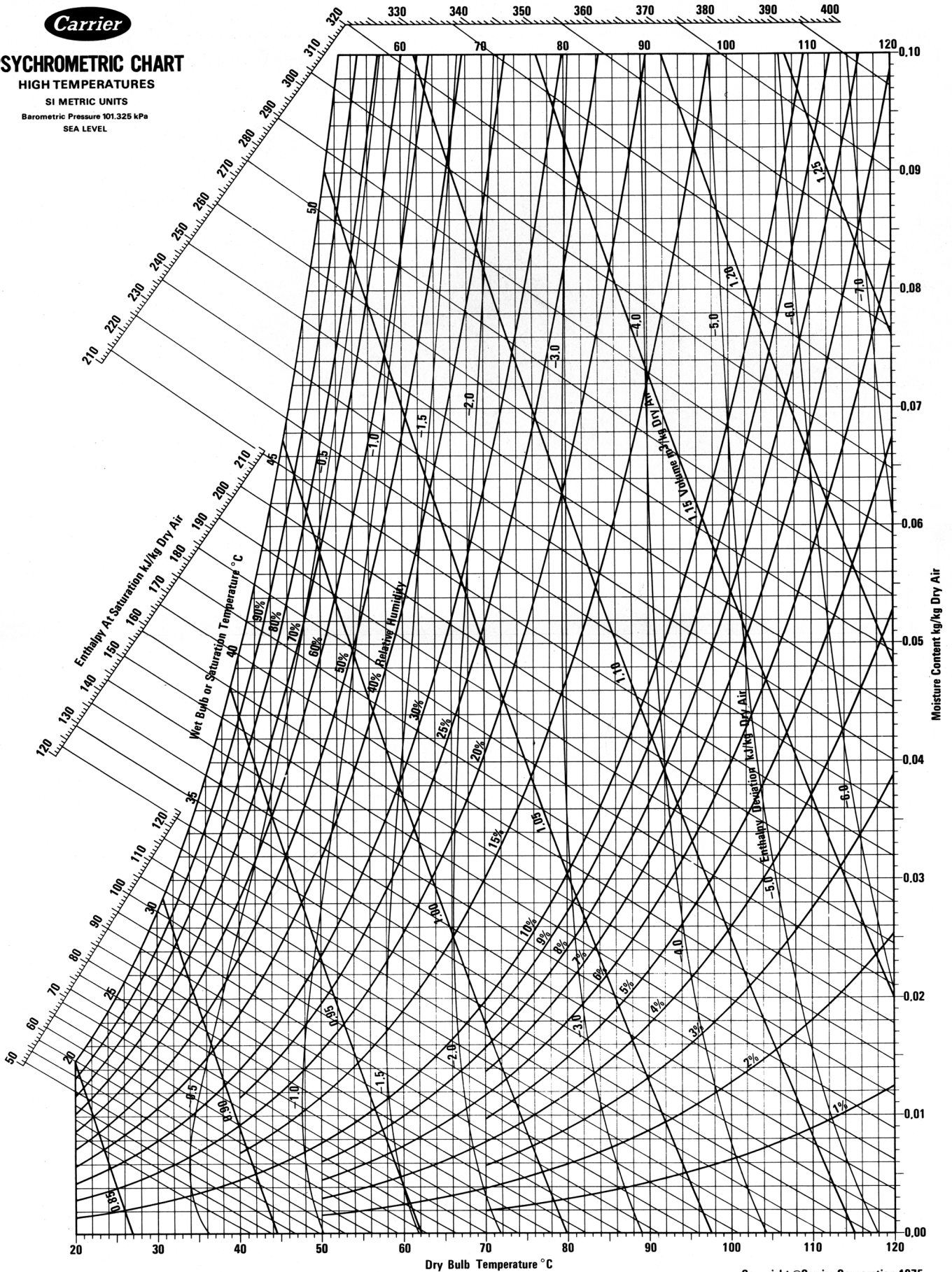
FIG. A.5. PSYCHROMETRIC CHART
